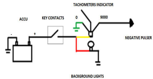
Fig. 3. Analog tachometer wiring
