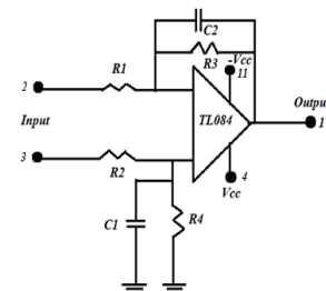
Fig.9. Voltage sensor using TL084 IC
