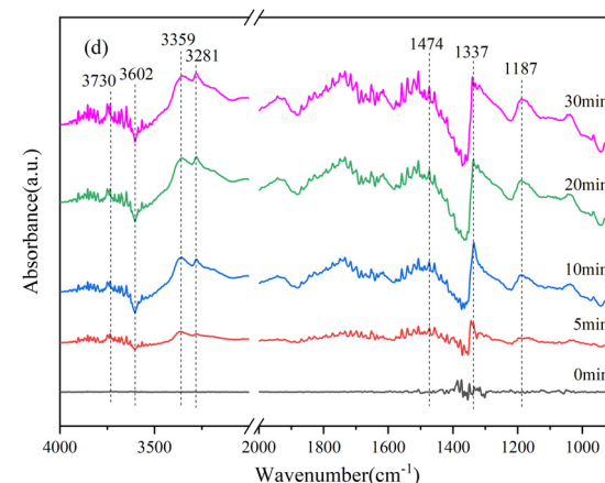
Figure 5. In-situ DRIFTS spectra of \text{NH}_3 adsorption. (a) Fe/ZSM-5, (b) Ce/ZSM-5, (c) 0.25\text{Ce-Fe/ZSM-5} , (d) 0.5\text{Ce-Fe/ZSM-5}
