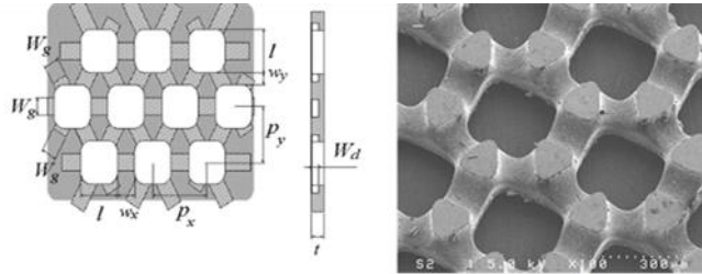
Fig. 2. Mesh sheet M1, M2, M3 and M4
