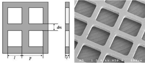
Fig. 3. Mesh sheet M5
