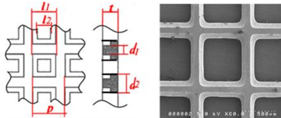
Fig. 4. Mesh sheet M7
