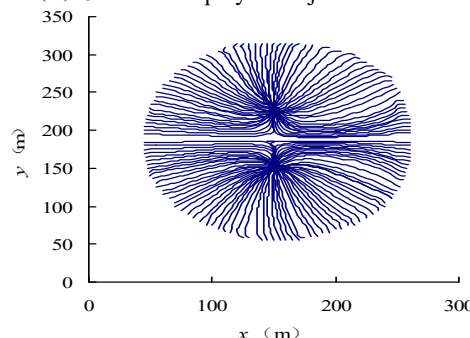
(d) 13 months of polymer injection in Juba well
