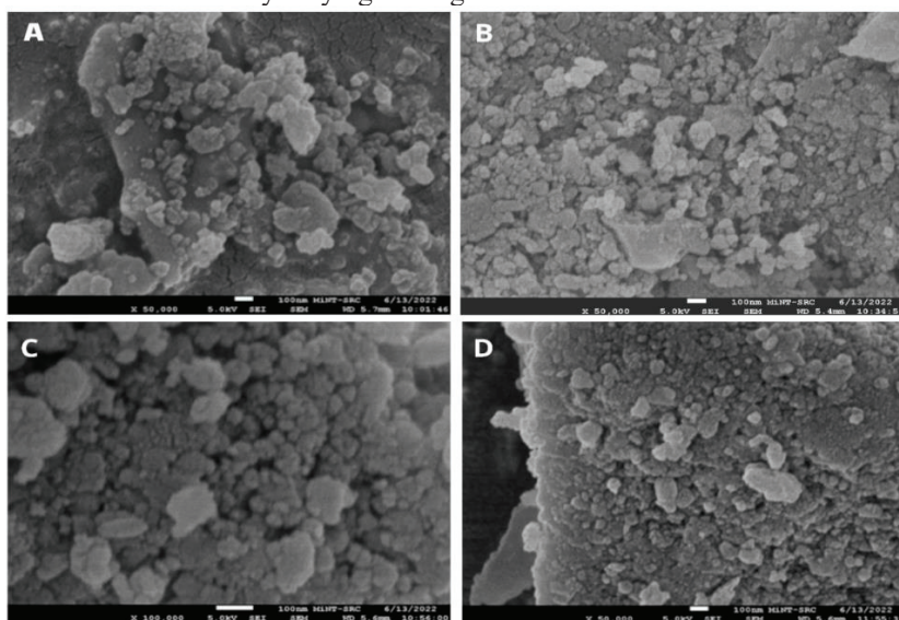
Fig. 7. nano RHA at milling time: (A) NS1, (B) NS2, (C) NS3, (D) NS4
